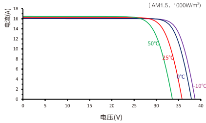
不同电池温度下, I-V 曲线图
