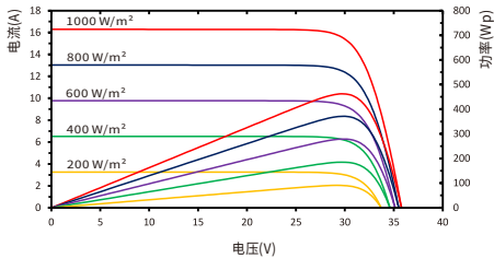
不同辐照度下, I-V 曲线图
